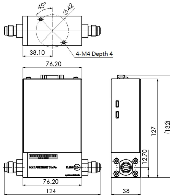
Рисунок 1. Габаритные размеры регулятора расхода газа
