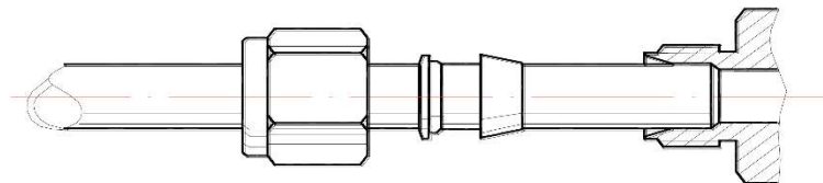
Рисунок 4. Зажимное соединение
