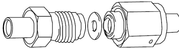
Рисунок 2. VCR со стандартным уплотнением
