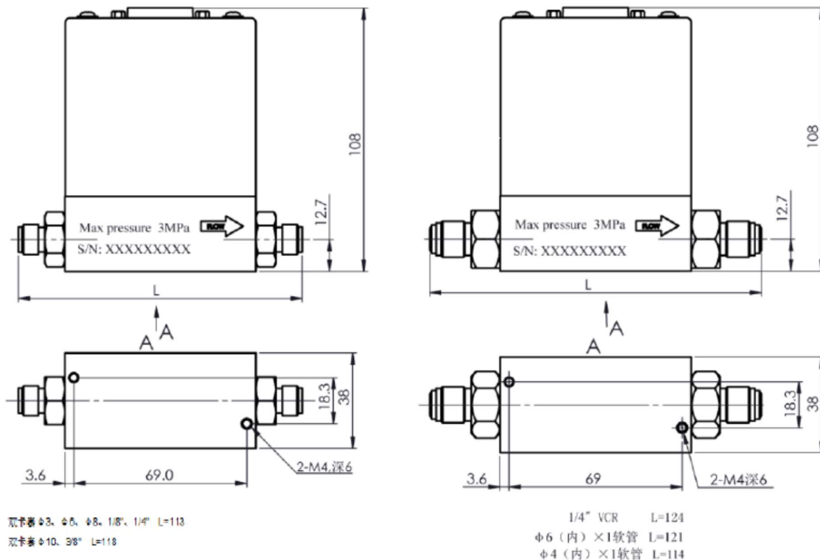
Рисунок 4. Габаритные размеры PPG D07-19B/BM
