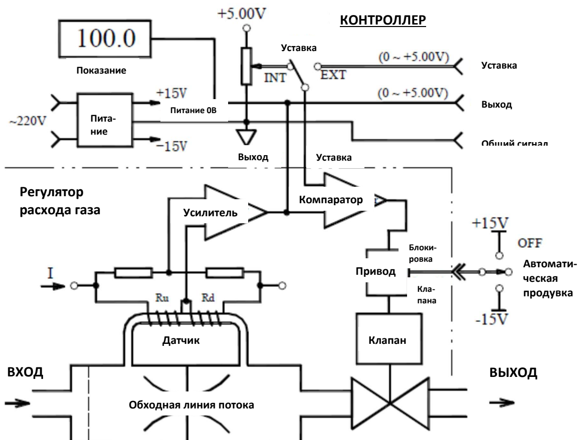
Рисунок 3. Принцип действия PPG D07-19B
