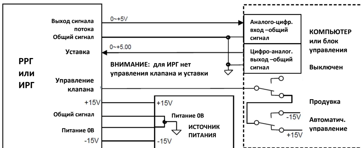
Рисунок 12. Подключение РРГ к компьютеру напрямую
