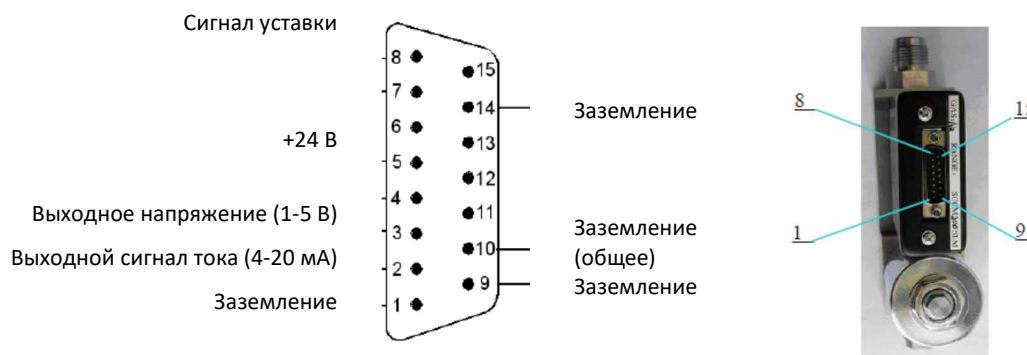
Рисунок 9. Электрический интерфейс ИРГ D07-23FM
