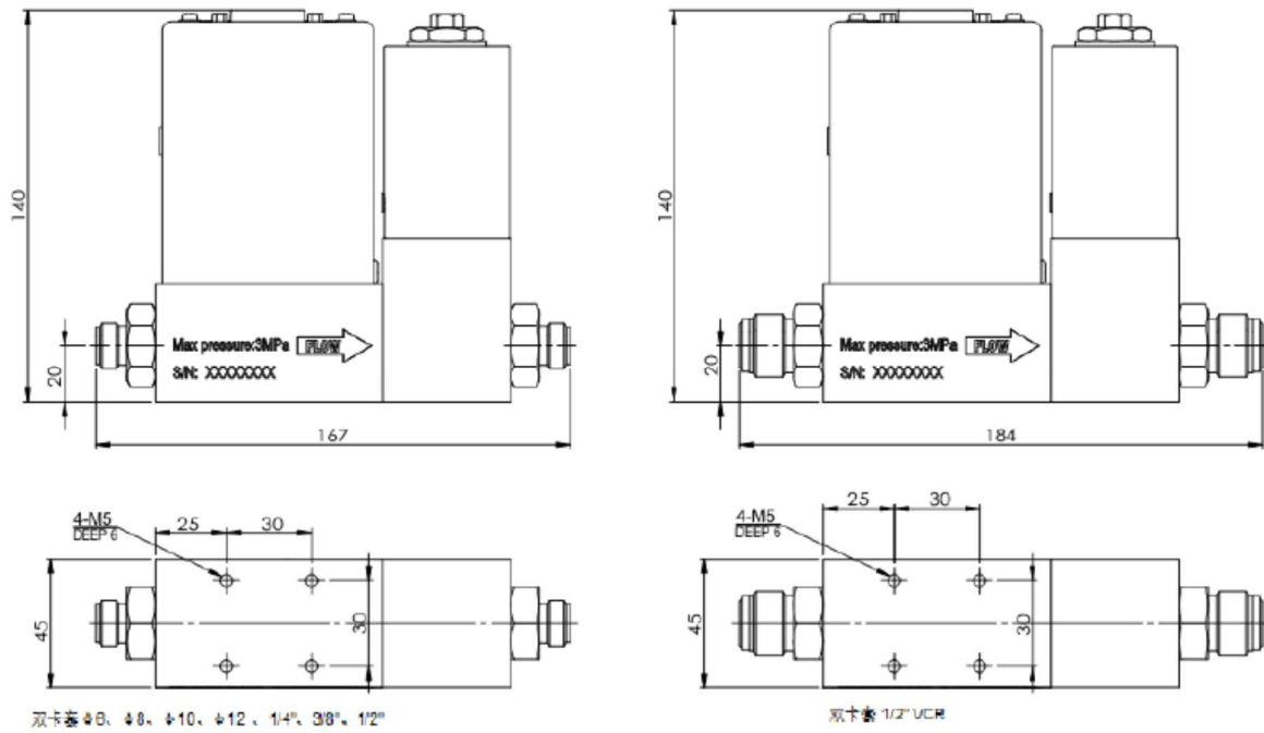
Рисунок 4. Габаритные размеры PPG D07-23F
