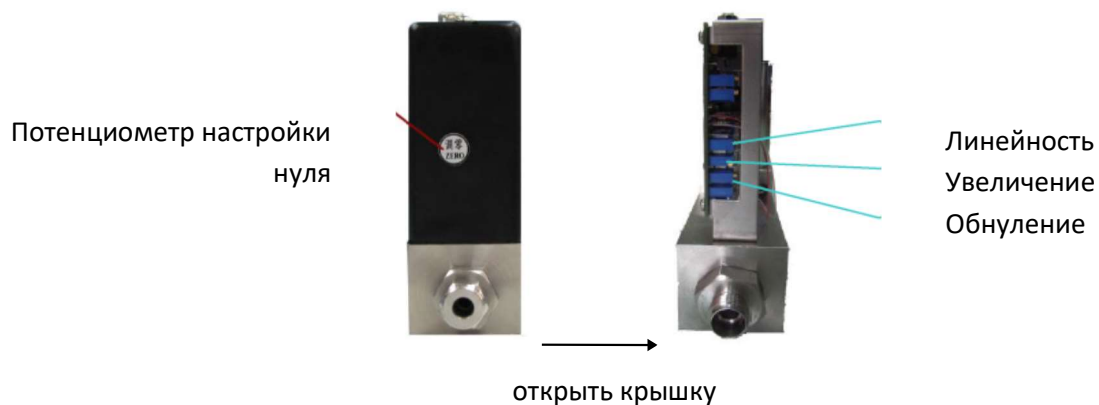
Рисунок 12. Расположение потенциометра нуля на D07-23F и D07-23FM
