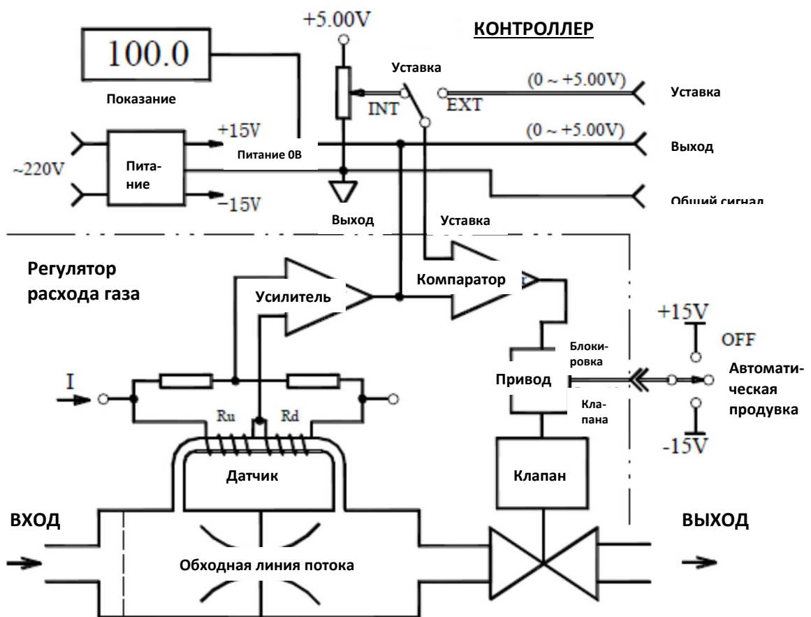
Рисунок 3. Принцип действия РРГ D07-23F
