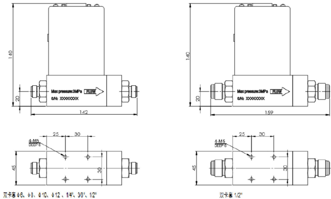
Рисунок 5. Габаритные размеры IPG D07-23FM
