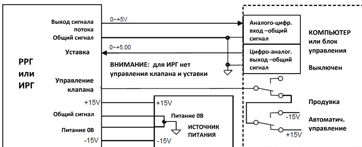
Рисунок 11. Подключение PPG к компьютеру напрямую
