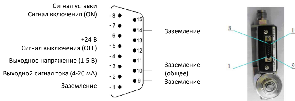
Рисунок 8. Электрический интерфейс РРГ D07-23F
