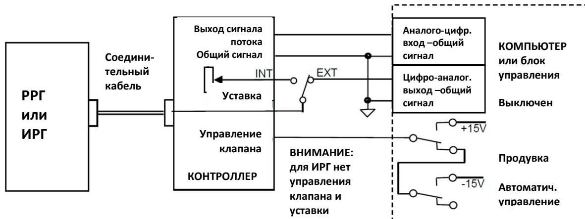
Рисунок 10. Подключение PPG к компьютеру через контроллер
